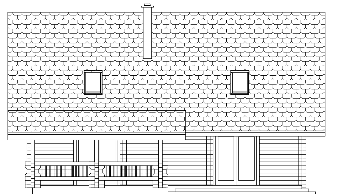
ELEWACJA TYLNA skala 1 : 100
